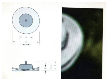
Bosch, Giampaolo Capobianco, "Un insolito e misterioso oggetto volante discoidale fotografato la sera del 19 giugno 2015." Elaborazioni
